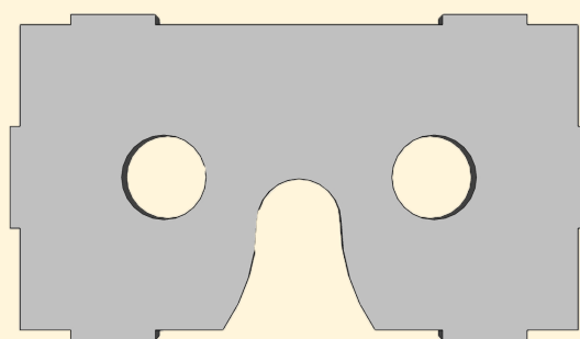
헤드셋 중간판
